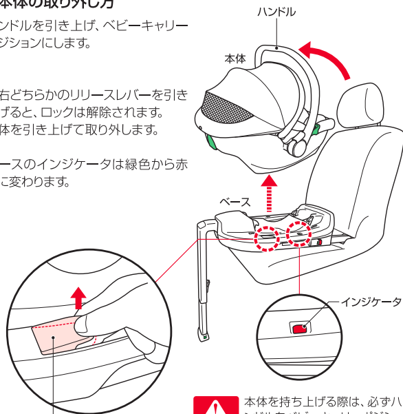
リリースレバー
